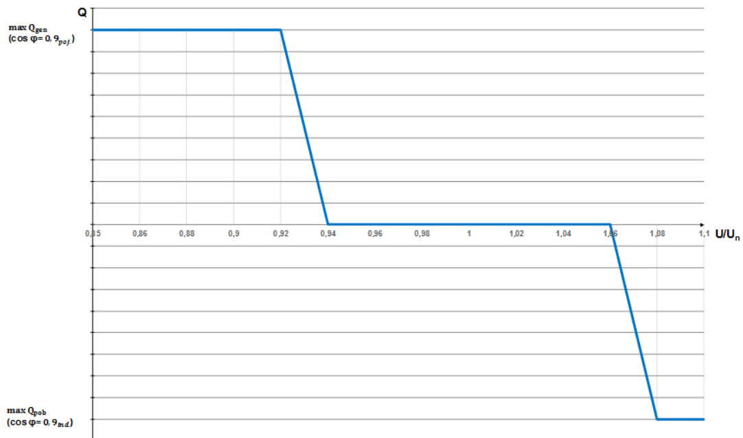
Rys. 3. Charakterystyka sterowania mocą bierną w funkcji napięcia wymagana przez TAURON Dystrybucja
